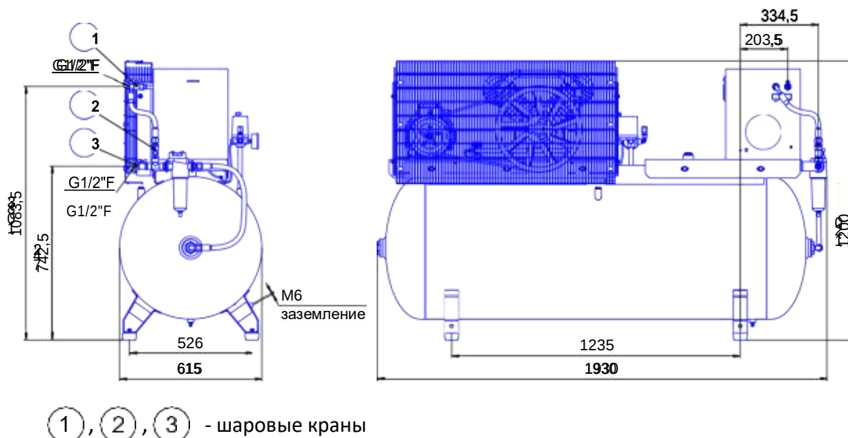
Рисунок 6 - Габаритные и присоединительные размеры компрессора СБ4/Ф-500.LB50Д
