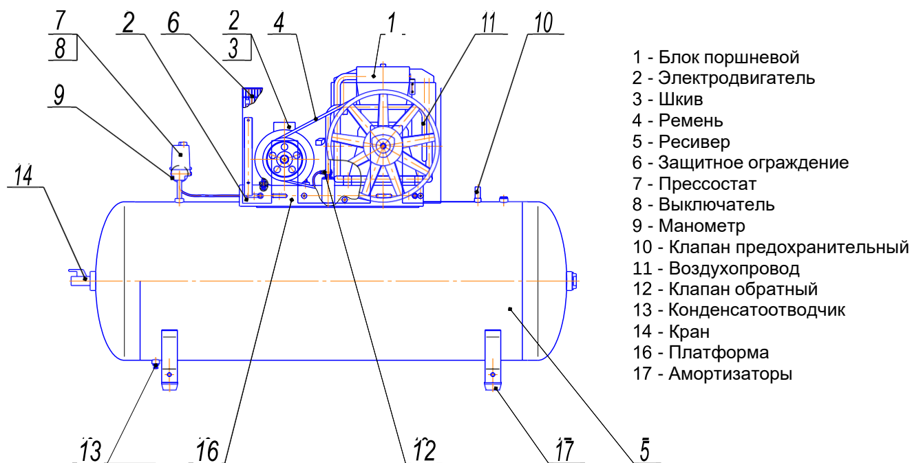
Рисунок 10 - Общий вид компрессора СБ4/Ф-500.АВ858/16
