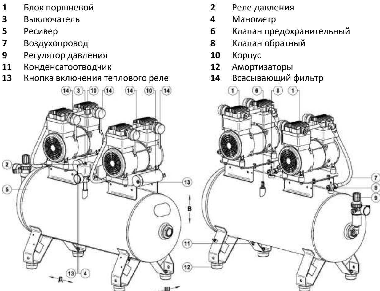
Рисунок 4 - Общий вид компрессора СБ4-100.OLD15Т
